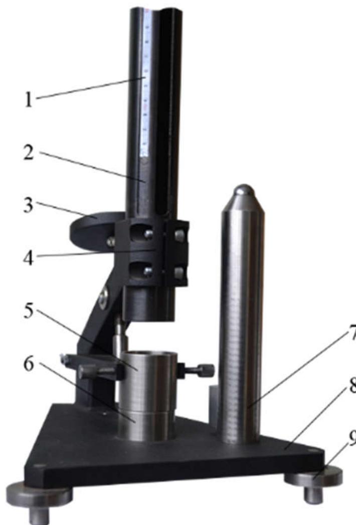
1 – шкала прибора; 2 – направляющая труба; 3 – механизм регулирования и фиксации образца контроля; 4 – фиксатор направляющей трубы; 5 – прижимная муфта; 6 – матрица; 7 – ударник (сферический боек); 8 – станина; 9 – регулятор положения станины.
